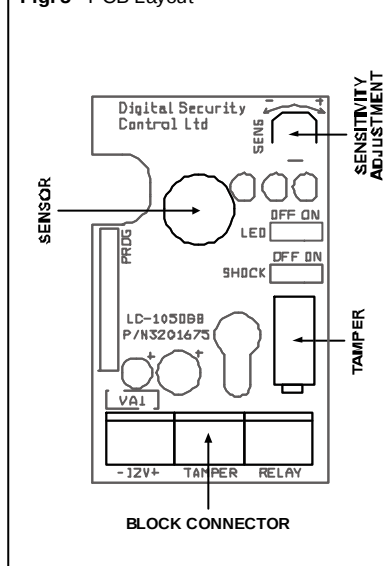
Fig. 5 - PCB Layout
